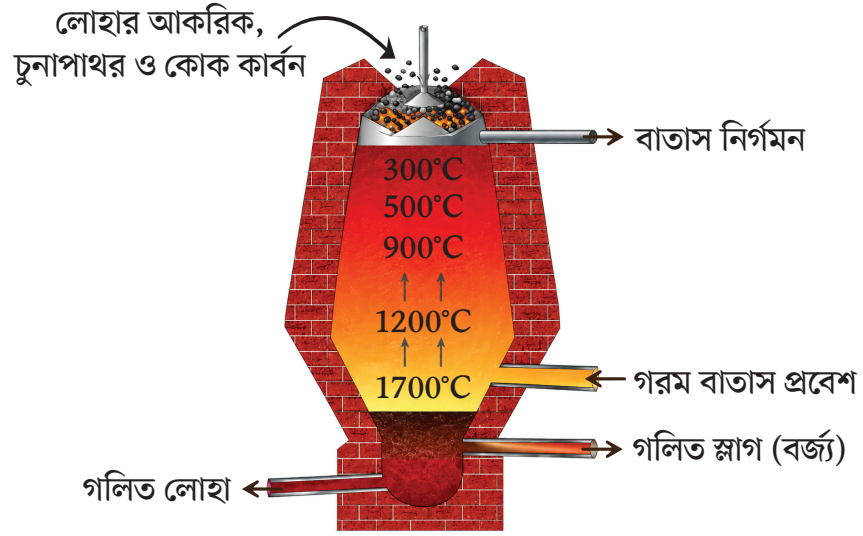
চিত্রঃ বাত্যাচুল্লিতে লোহা উৎপাদনে কোক কার্বনের ব্যবহার
